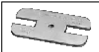
Měřítka pro kontrolu výšky Obj.č. 230495-1 Používá se pro kontrolu správného stisknutí lisovacích konektorů
