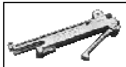
Nástroj pro TUS verze Obj.č. 230722-1 Nástroj má již výškové měřítka pro kontrolu správného slisování dle výšky konektoru
